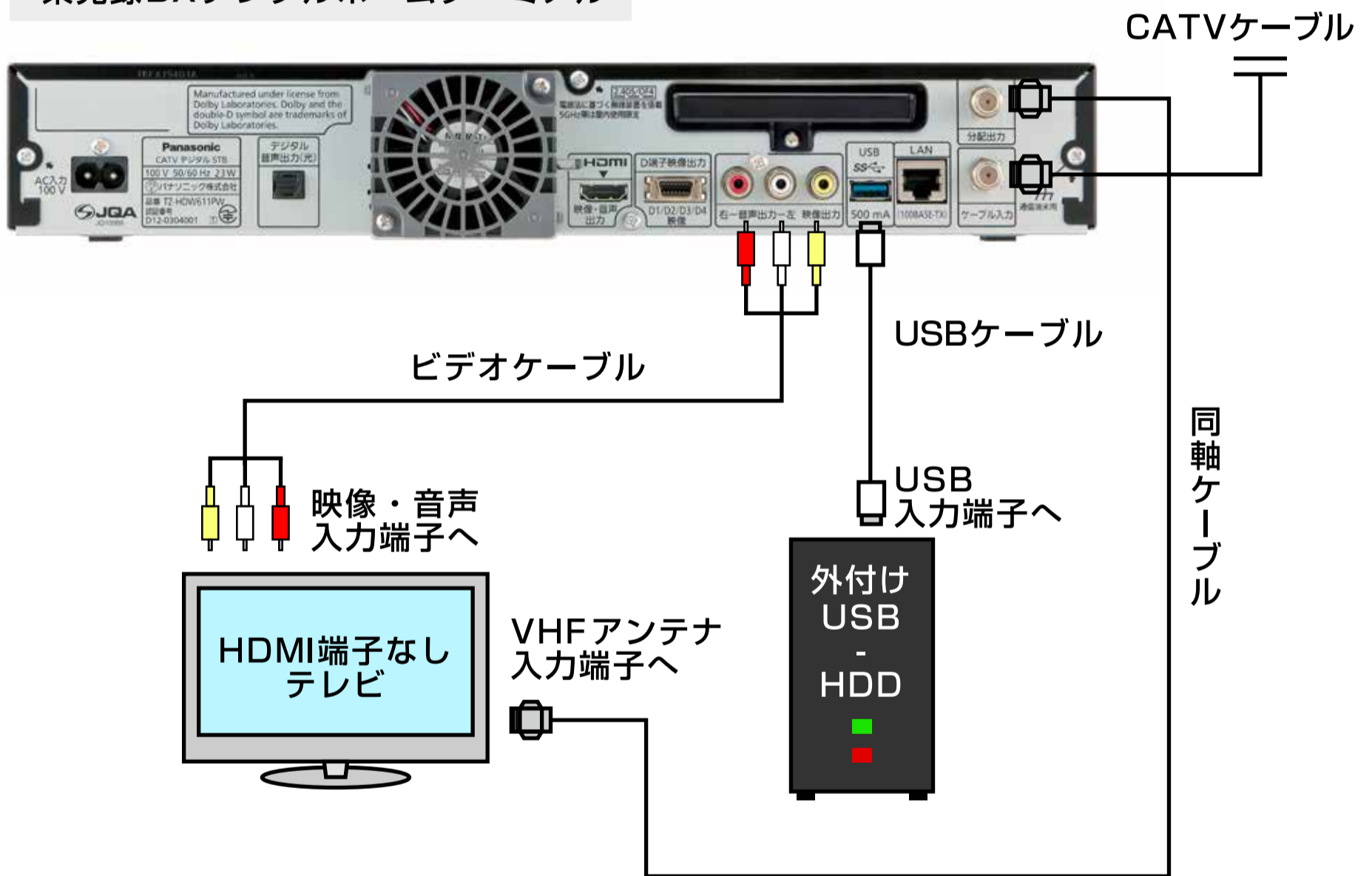
楽見録DXデジタルホームターミナル
